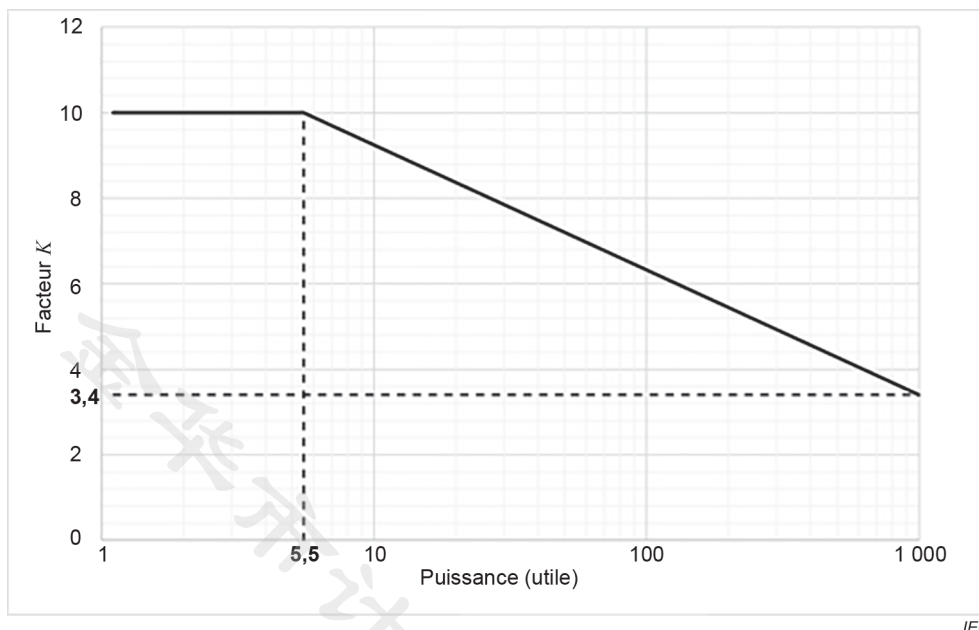
Figure 13 – Facteur K pour déterminer R_{PE,M}
